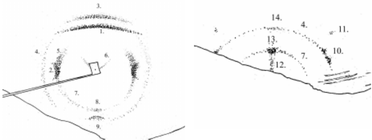
Kuva no 126: Kaksi vaihetta Lascarin outojen halojen näytelmästä 27/28.11.1997. 1. 23^{\circ} ylempi parheelia, 2. 18^{\circ} parheeliat, 3. “Scheinerin halon ylläsivuava kaari”, 4. 28^{\circ} rengas eli mahdollinen Scheinerin halo, 5. n. 19^{\circ} “sivuava kaari”, 6. pyramidiaurinkokaari, 7. 18^{\circ} rengas, 8. n. 19^{\circ} “alläsivuava kaari”, 9. 20^{\circ} alempi parheelia, 10. “Scheinerin halon” ylempi lateraali-kirkastuma, 11. 35^{\circ} ylempi parheelia, 12. auringonpilari, 13. 20^{\circ} ylempi parheelia, 14. “Scheinerin halon” toinen “ylläsivuava kaari”.
