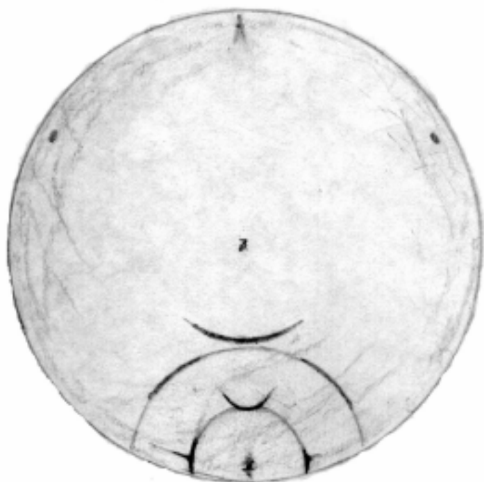
Kuva no 110: Hienosti kehittynyt halonäytelmä 10.5.1988 Joensuun taivaalla Marko Riikosen havaitsemana. Toukokuun kymmenennen päivän multihalo näkyi myös Kuopiossa, jossa sitä seurasivat Juhana Hakumäki ja Timo Nousiainen. Molempien kaupunkien havaintoraporteissa vastapuolen ilmiön todettiin olleen hyvin diffuusin epämääräinen. Kuvassa näkyvät pitkulaiset kirkastumat 46^\circ renkaalla ovat 46^\circ ylläsiuvaavan maksimi-intensiteetin kohtia.
