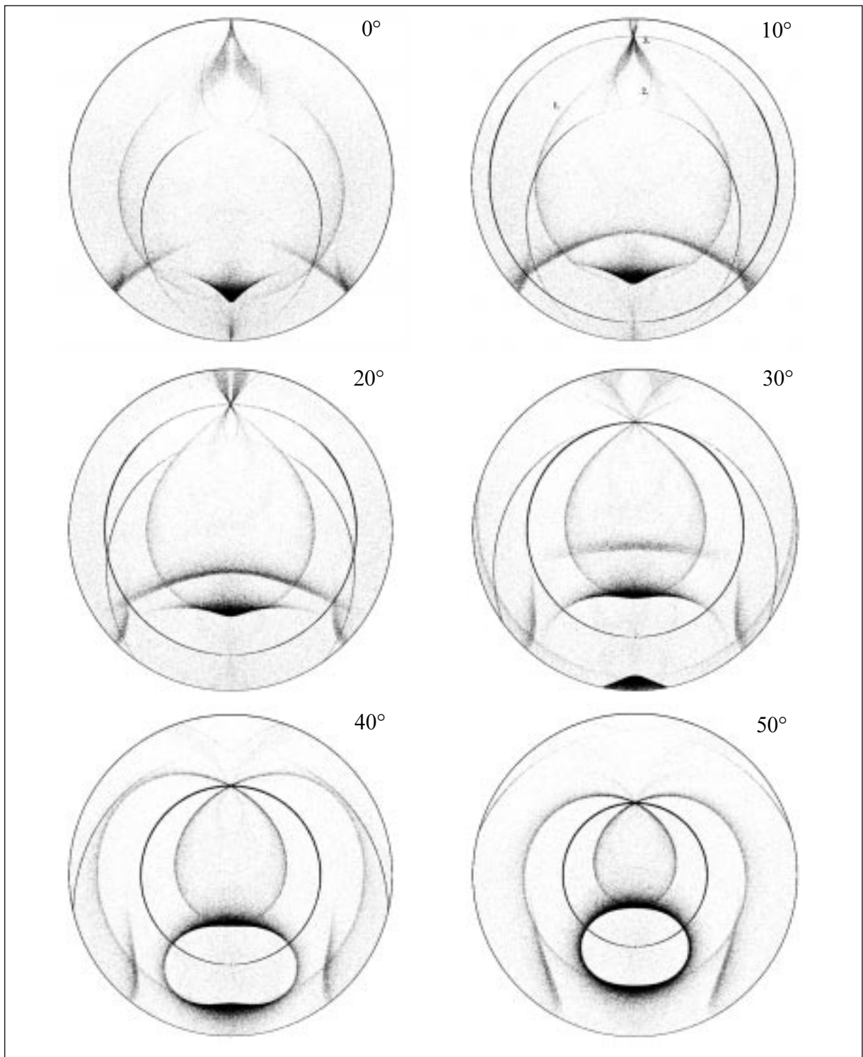
Kuva no 105: Simulaatiot kaikista sivuava-asentoisen pylväskiteen aiheuttamista haloista. Kide putoaa pääakseli vaakasuorassa, mutta on vapaa pyörimään pääakselin sekä pystyakselin ympäri. Wegenerin vasta-aurinkokaaret sivuavat 22^\circ sivuavia kaaria. Vasta-aurinkopisteeseen kaaret yltävät yli 20^\circ aurinkokorkeuksilla. Tätä suuremmilla Auringon korkeuksilla kaaret muodostavat suljetun lenkin sivuten 22^\circ yllä- ja allasivuavia ja kulkien vasta-aurinkopisteen kautta. 1. Wegenerin vasta-aurinkokaaret, 2. Trickerin vasta-aurinkokaaret, 3. Greenlerin diffuusit vasta-aurinkokaaret.
